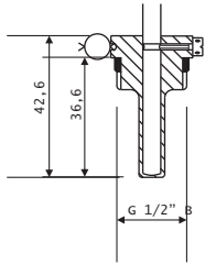
Рис. 1 Втулка термометра сопротивления (ТСП)
